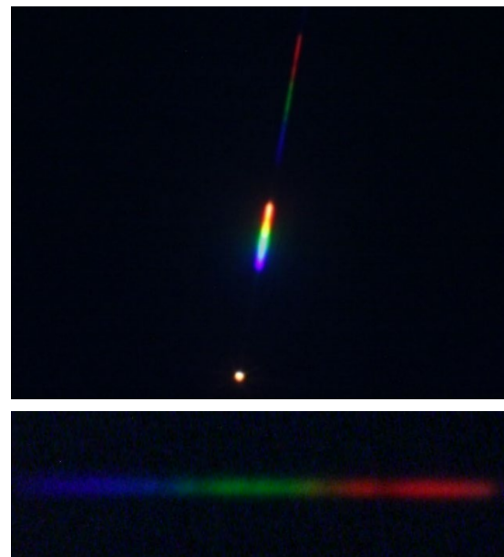
Slika 1: Osnovna in obrezana slika spektra Betelgeze
